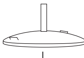
Betonsockel mit Henkel ø 66 cm, 50 kg
